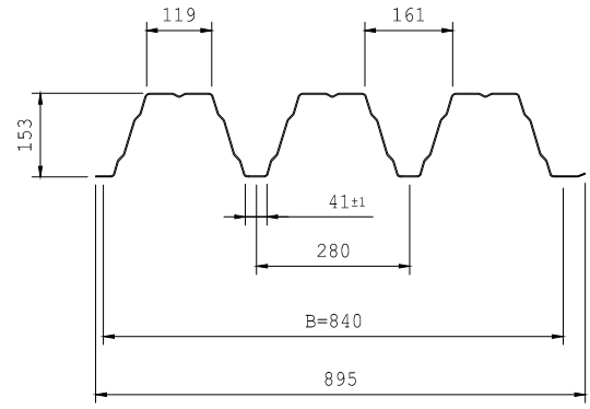
DF H153-840
