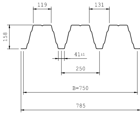
DF H158-750
