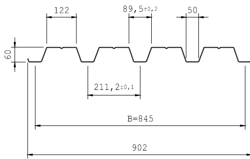
DF H60-845
