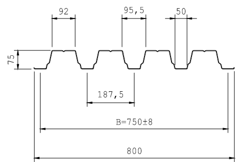
DF H75-750
