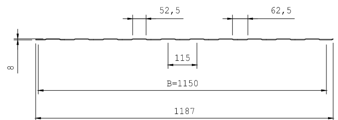
DF C8-1150
