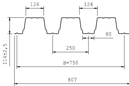
DF H114-750
